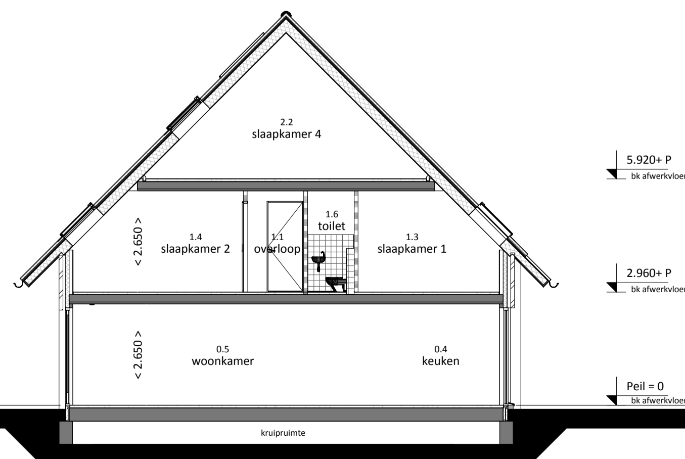
- doorsnede bouwnr. 3, 4, 5 en 9 -
