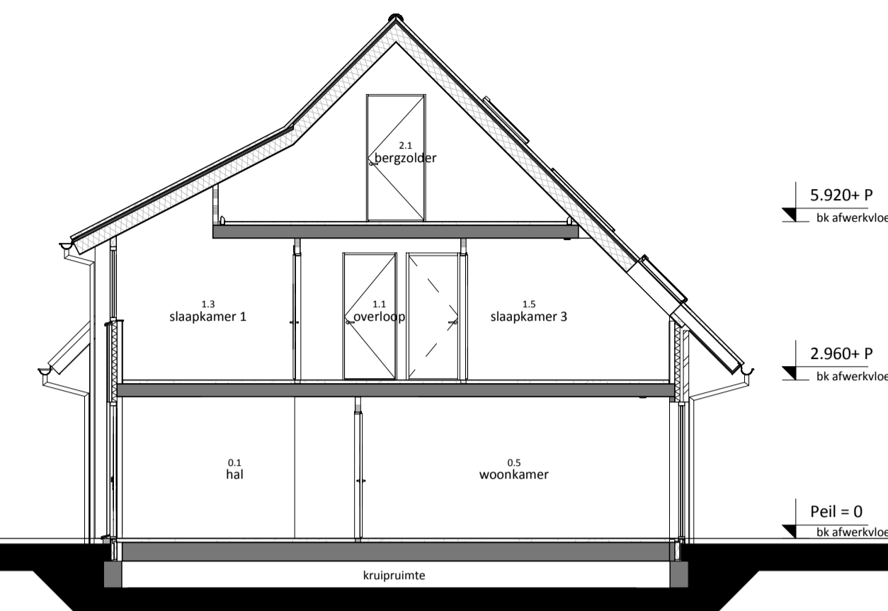
- doorsnede bouwnummer 17 en 18 -
