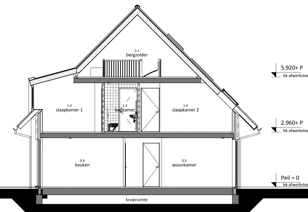
- doorsnede bouwnummer 14, 15 en 16 -
